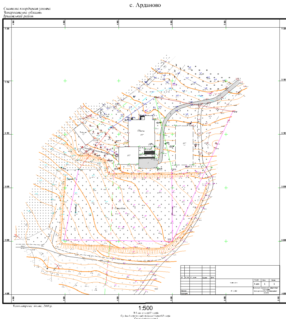
Рис.1 .План тахеометричного знімання.
